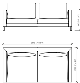
DIVANO 2 POSTI / 2-SEATER SOFA_214X107
