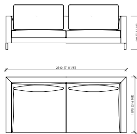
DIVANO 2 POSTI / 2-SEATER SOFA_234X107
