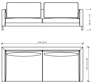
DIVANO 2 POSTI / 2-SEATER SOFA_254X107
